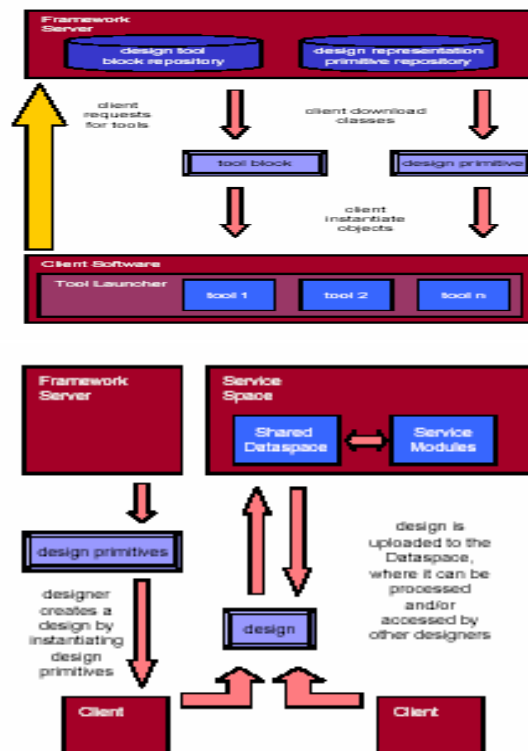
Fig. 1.- Framework server concept.
